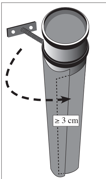
4 Sovrapporre senza lasciare spazi / Overlap taking care not to leave gaps / Bei der Umwicklung auf eine lückenlose Überlappung achten / Lors du recouvrement ne pas laisser d'espaces, faire chevaucher le matériel
