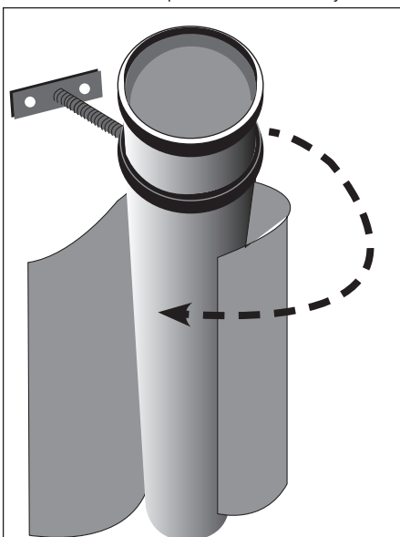
3 Ricoprire il tubo con il lato in PU verso l'interno / Wrap around the pipe with PU foam inside Umwickeln Sie das Rohr mit der PU-Schaumseite innenlegend / Enroulez-le autour du tuyau avec de la mousse PU à l'intérieur
