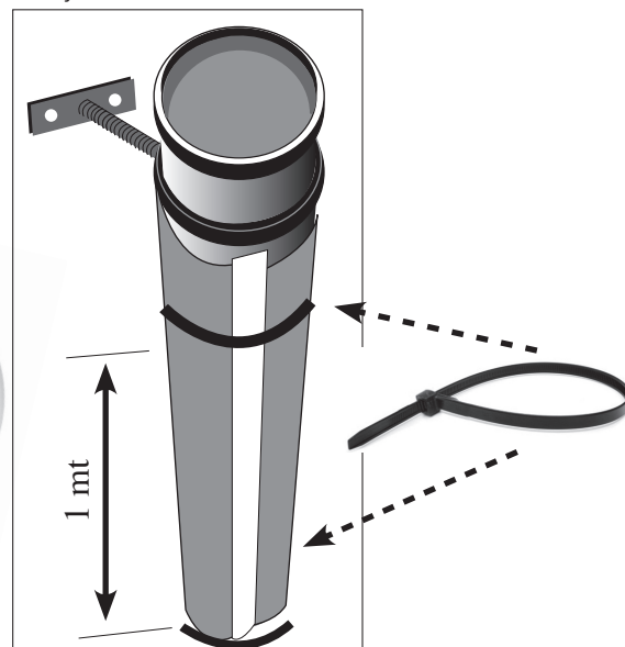
6 Fissare infine con fascette, lasciando uno spazio di circa 1 mt / Finally fix with cable ties. Correct applications of ties is 1 meter / Zum Schluß mit Kabelbinder fixieren / Der richtige Abstand der Kabelbinder beträgt 1meter / Enfin fixer avec des colliers de serrage. L'application correcte de liens est de 1 mètre
