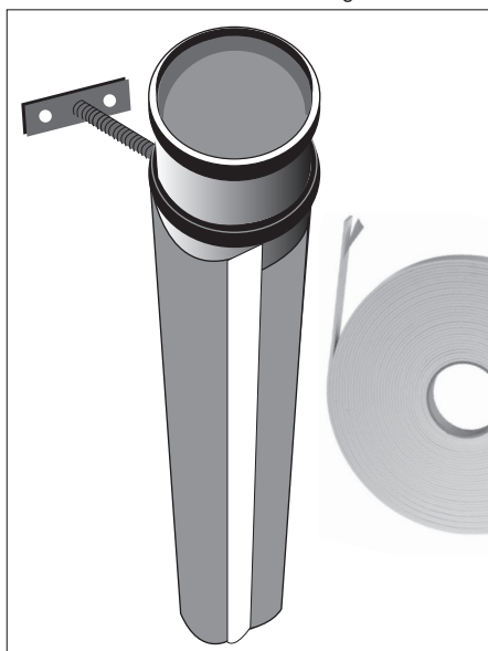
5 Sigillare la chiusura verticale con una guarnizione in PE / Seal the vertical side using PE Gaskets / Dichten Sie die vertikale Fuge mit einen PE Dichtungsbund ab / Sceller le côté vertical en utilisant des joints PE
